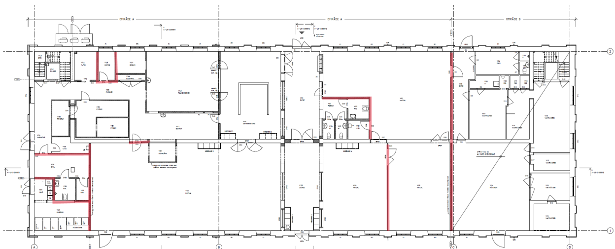
Figur 1: Markerade väggar där krav på luftljudsisolering ska uppfyllas.
